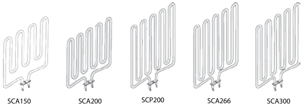
Рис. 4 Fig. 4 ТЭН Heating Elements
