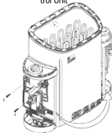
Рис. 5B | Перестановка встроенного Fig. 5B | блока управления Repositioning the Built-in-Con- trol Unit
