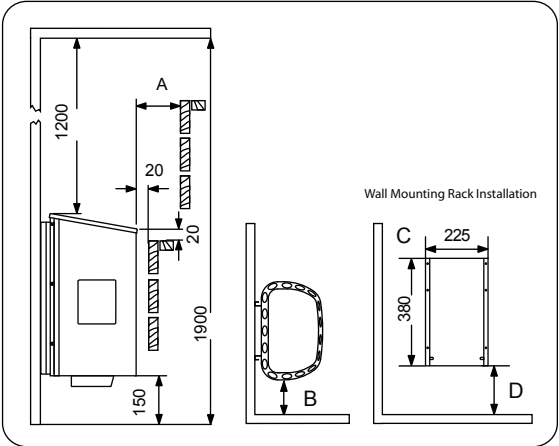
Рис. 1 | Минимальные расстояния безопасности(mm) Fig. 1 | Minimum Safety Distance (mm)
