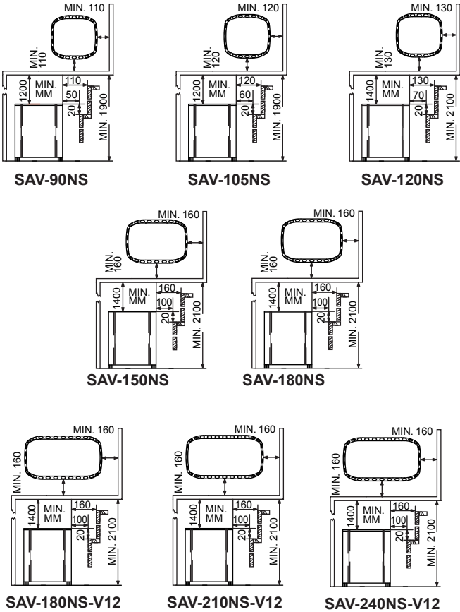
Рис 2 Fig. 2 Минимальные безопасные расстояния (mm) Minimum safety distances (mm)
