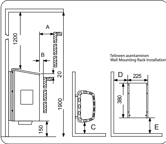
Рис. 1 Минимальные расстояния безопасности(mm) Fig. 1 Minimum Safety Distance (mm)
