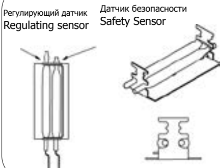
Расположение датчиков печей NB Sensor location NB-heaters
