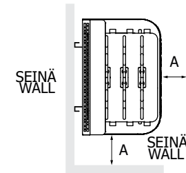
YLÄNÄKYMÄ TOP VIEW
