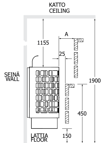
SIIVUNÄKYMÄ SIDE VIEW
