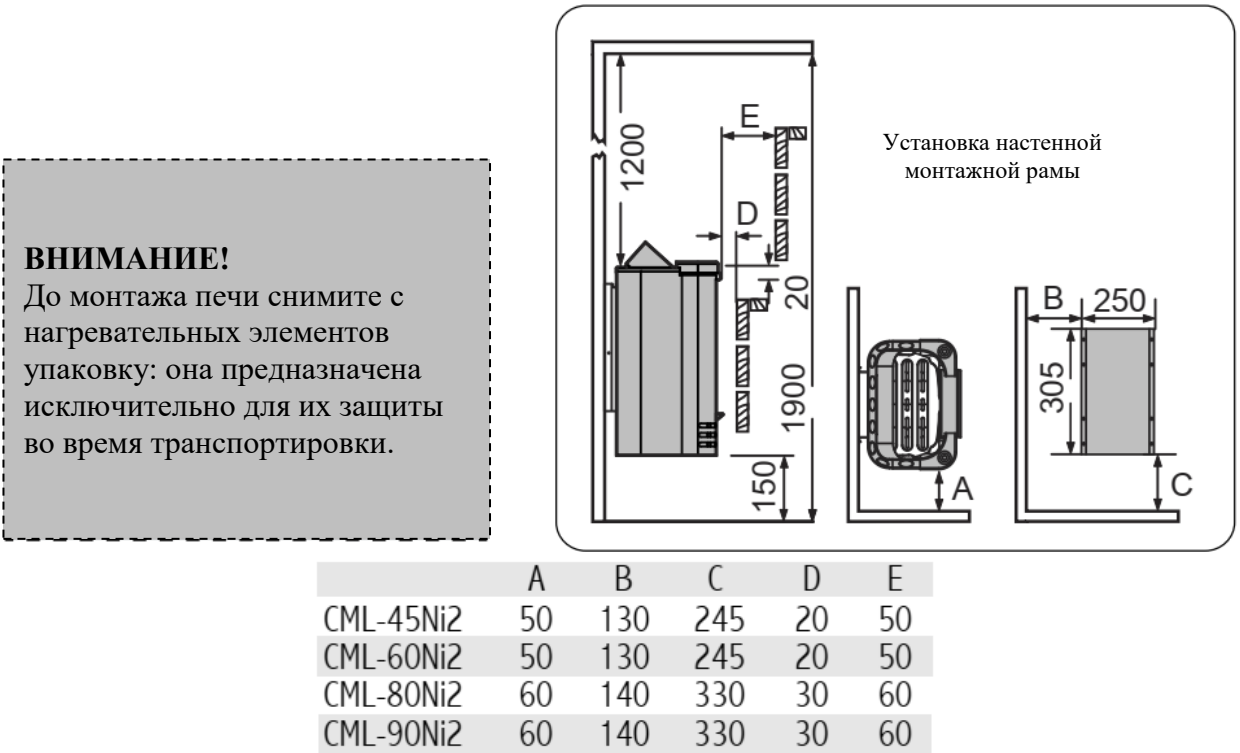
Рис. 1. Минимальные безопасные расстояния (мм)
